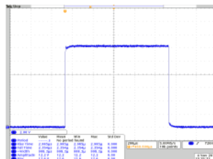
50A, コンプライアンス電圧 24V, 20Hz, パルス幅 1,000us
