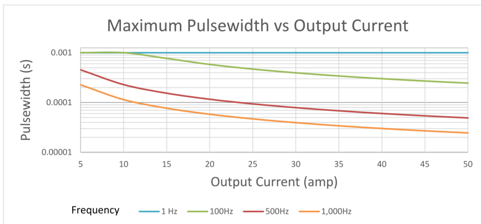
最大パルス幅対 出力電流
