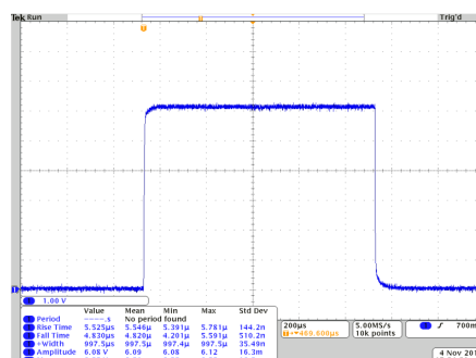
25A, コンプライアンス電圧 18V, 20Hz, パルス幅 1,000us
