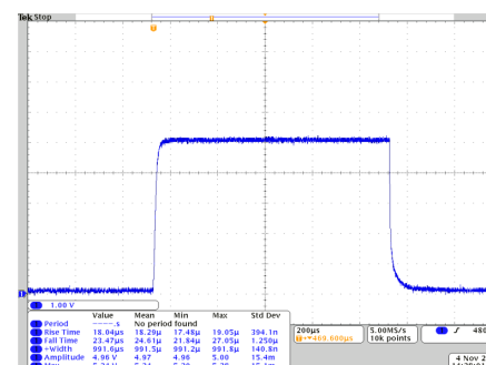
5A, コンプライアンス電圧 17V, 20Hz, パルス幅 1,000us
