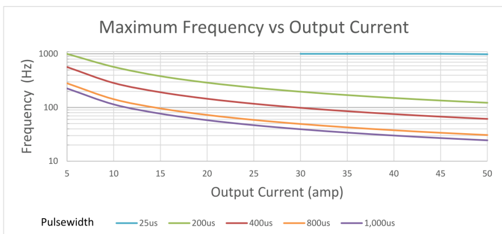
最大周波数対 出力電流
