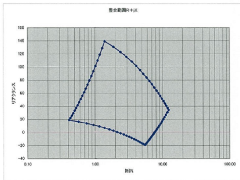
整合範囲 (R + j X) 表記
